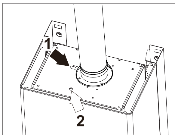
Рис.12 Точки подключения газоанализатора
