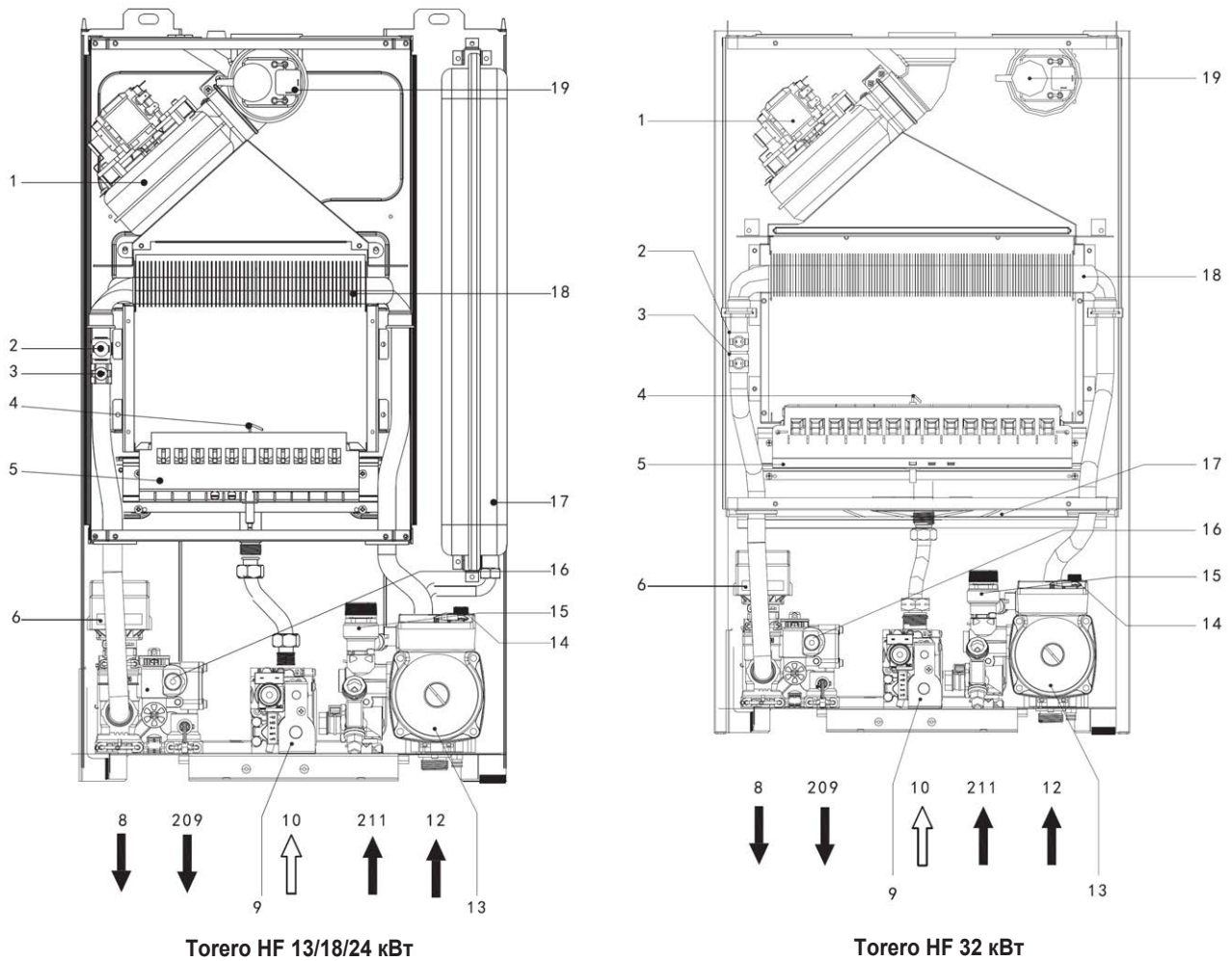
Рис.14 Конструкция котла
