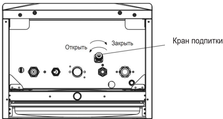
Рис.3 Кран подпитки
