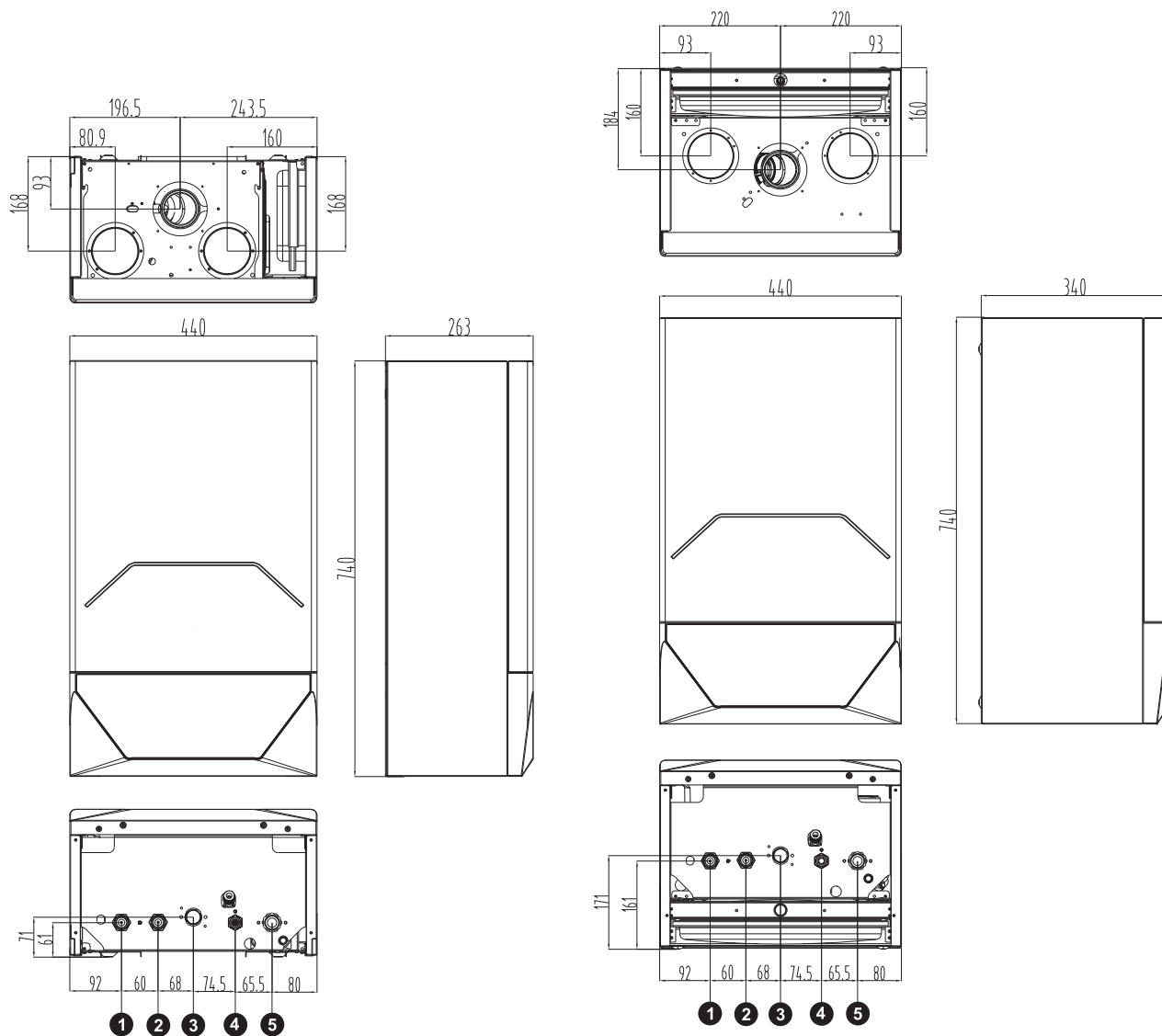
Размеры котла Torero HF 13-24 кВт
