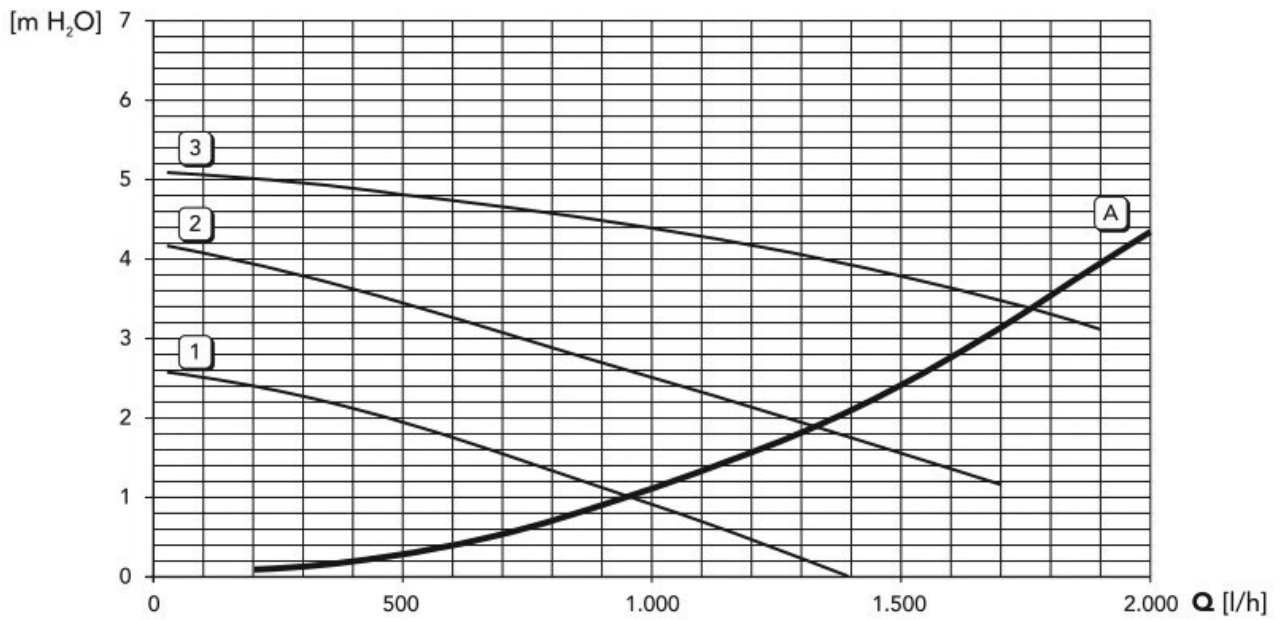
Рис.16 Диаграммы давление-мощность
