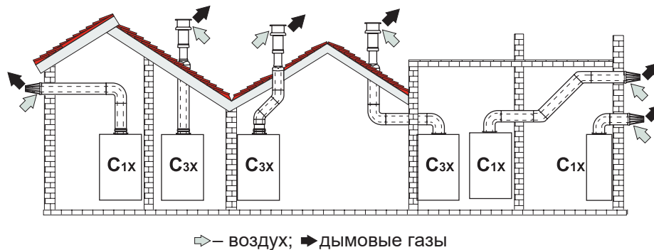
Рис.8 Примеры присоединения с помощью коаксиальных труб
