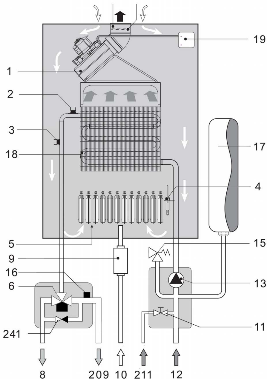
Рис.15 Гидравлическая схема
