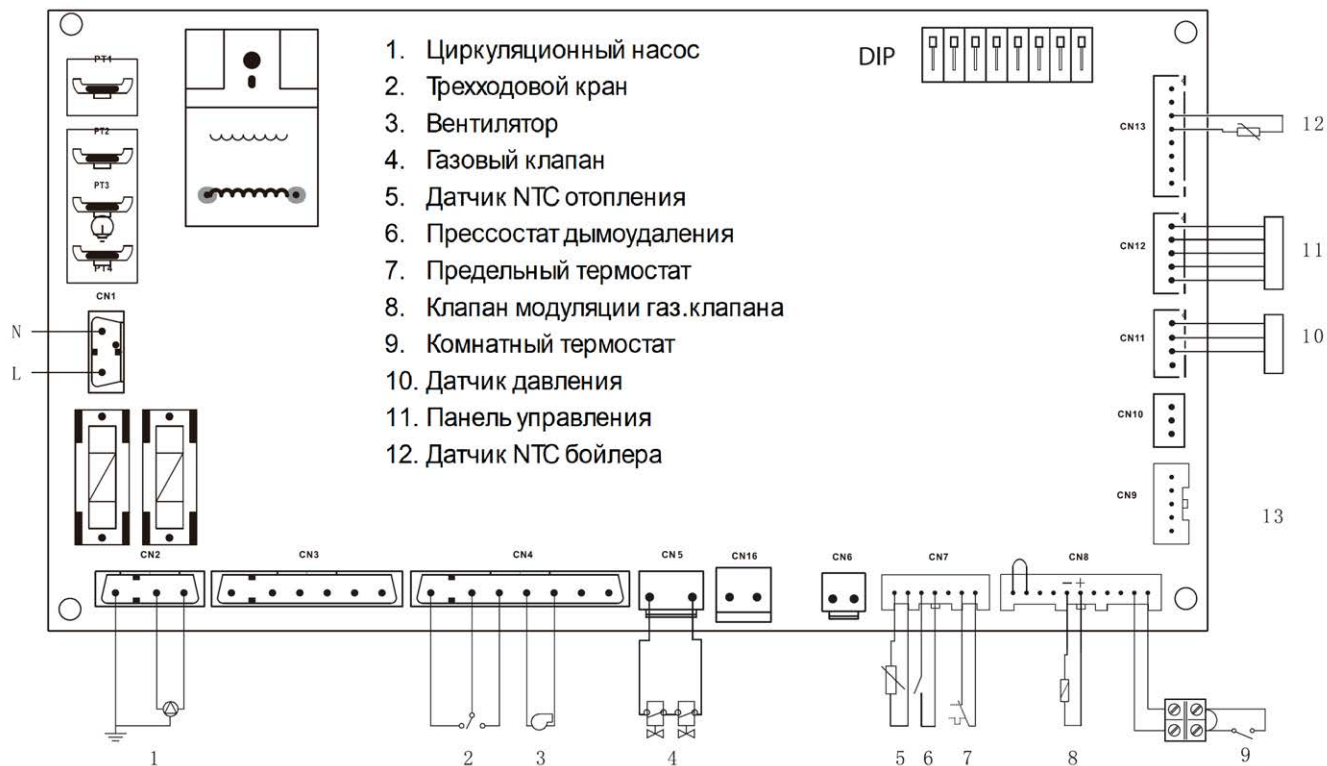
Рис.19 Электрическая схема
