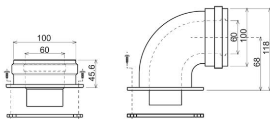
Рис.9 Начальные элементы для коаксиальных воздуховодов
