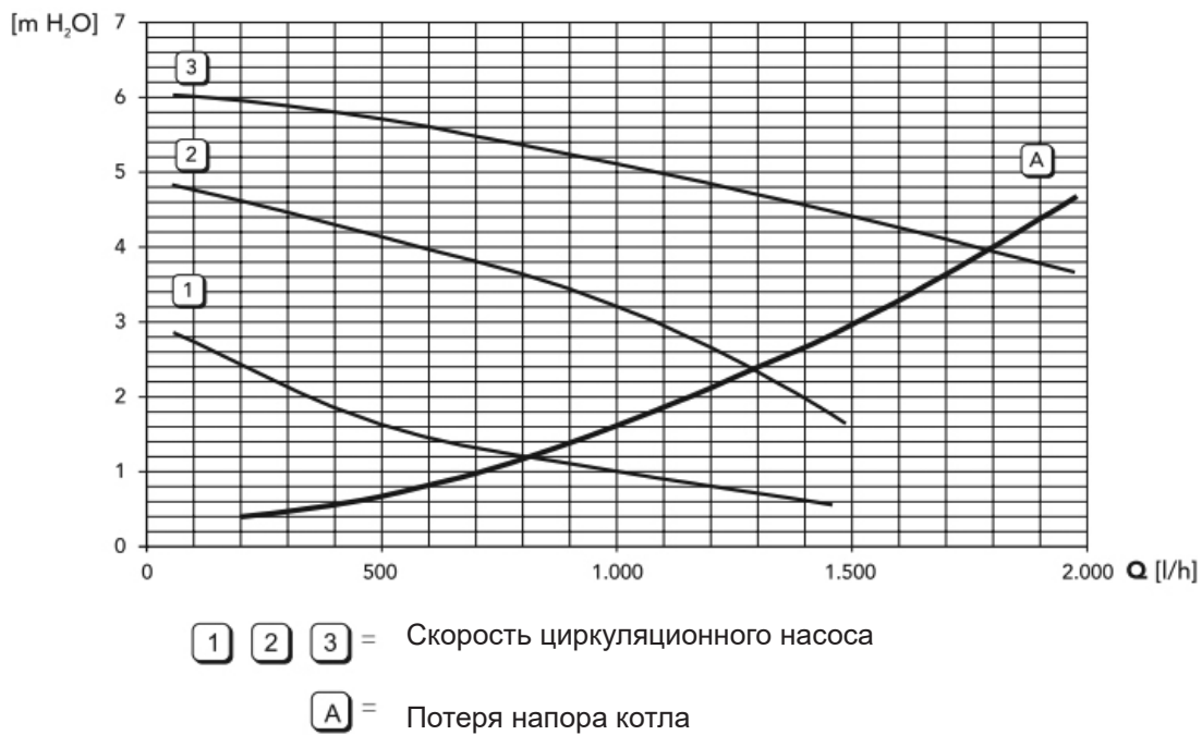
Рис.18 Производительность и напор циркуляционного насоса (32 кВт)
