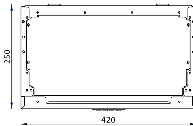
Рис. 12. Вид сверху
