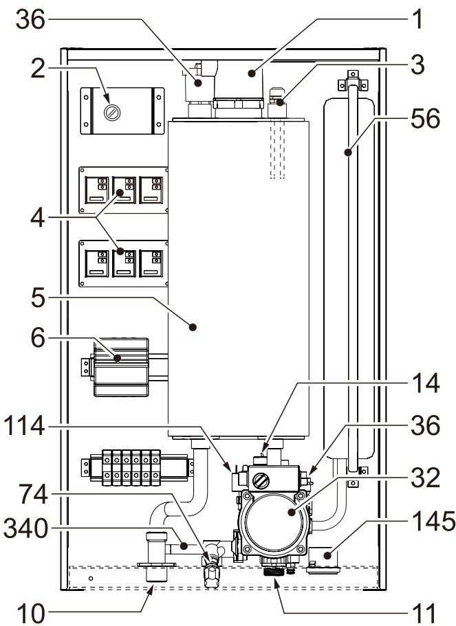
Рис. 14. SIRIO 15-24 кВт
