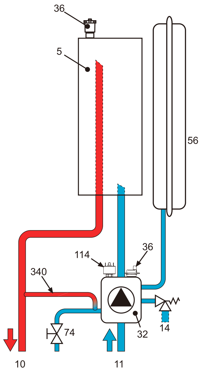
Рис.15 Гидравлическая схема
