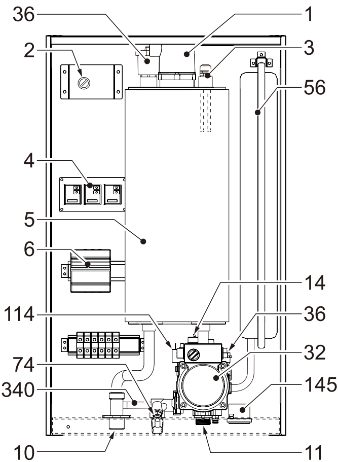
Рис. 13. SIRIO 6-12 кВт
