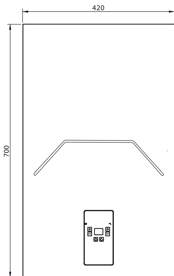
Рис. 9. Вид спереди
