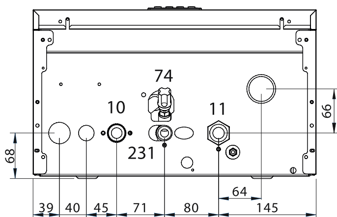
Рис. 11. Вид снизу
