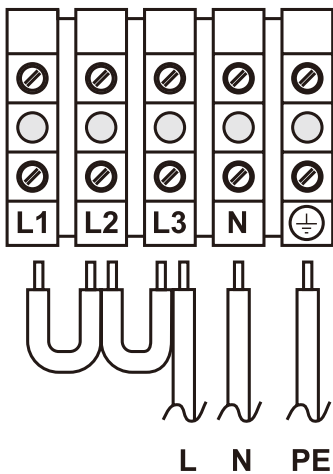
Рис. 19. Однофазная проводка
