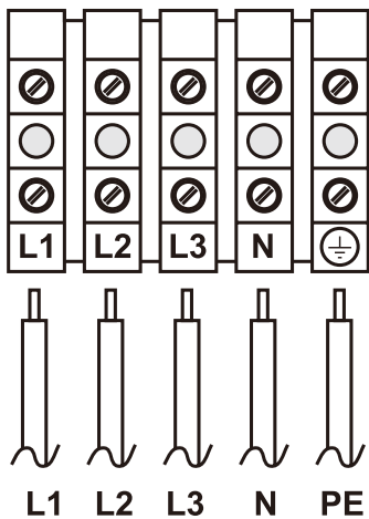
Рис. 18. Трехфазная проводка
