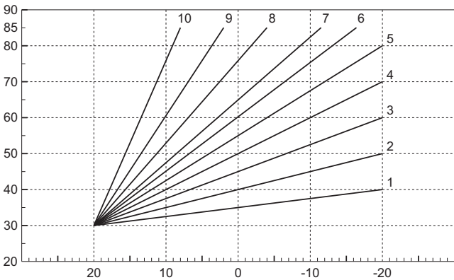
рис. 31- Компенсационные кривые
