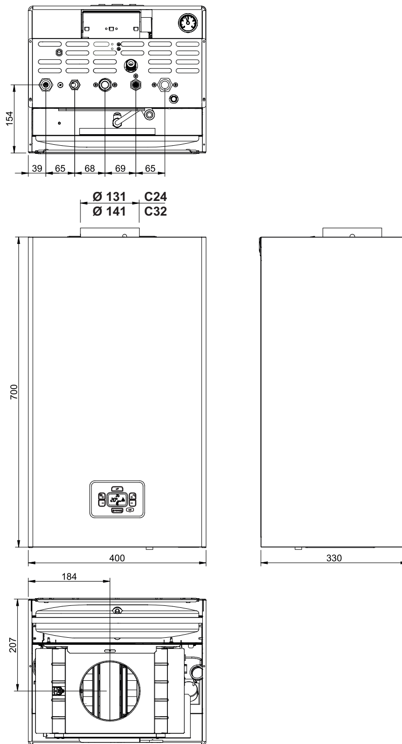
рис. 15- Размеры и соединения
