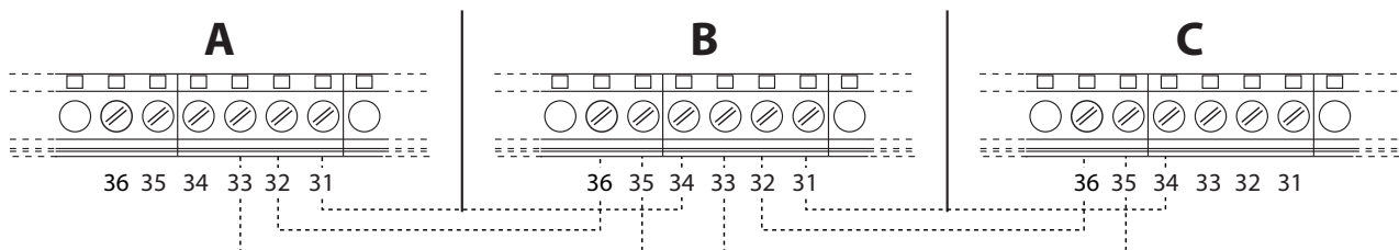
рис. 56- Каскадное подключение
