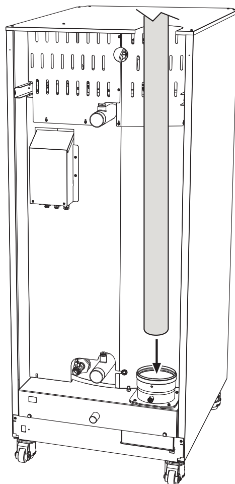
рис. 57- Выход дымов
