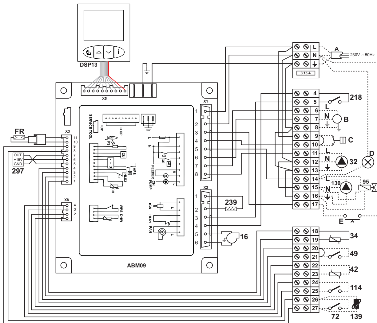
рис. 17 - Электрическая схема
