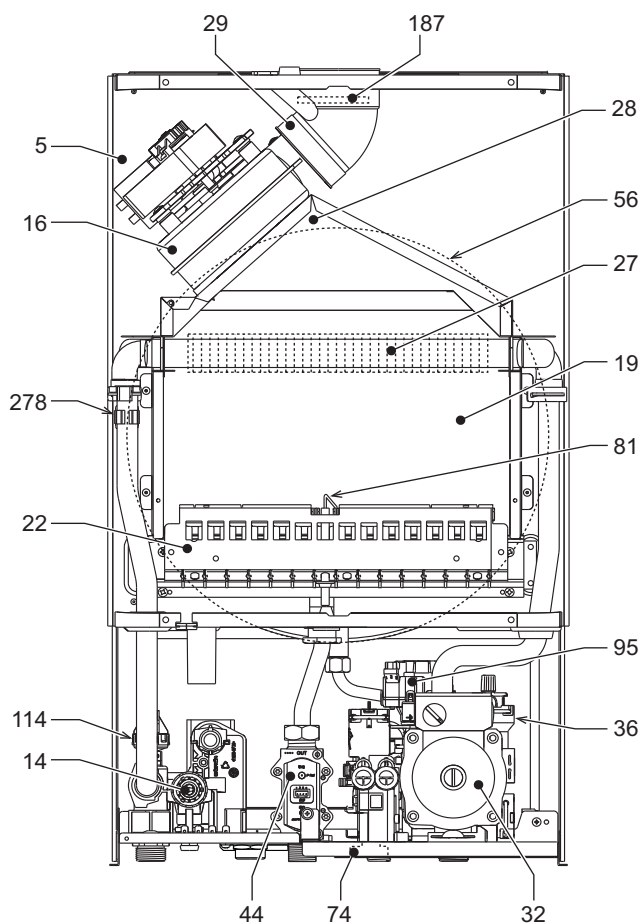
рис. 28- Общий вид - FL D HF32
