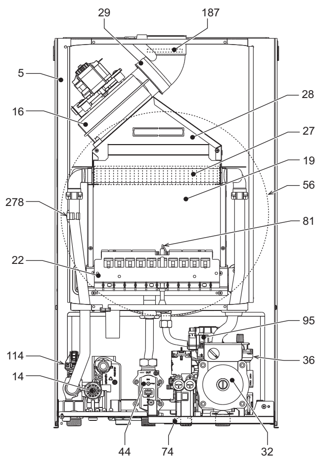
рис. 27- Общий вид - FL D HF24
