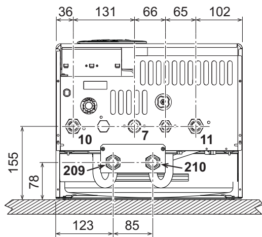
рис. 25- Вид снизу - HF24 и HF32
