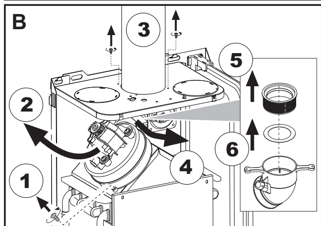
A Замена диафрагмы в не установленном котле
