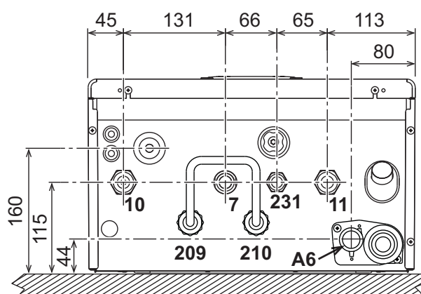
рис. 52- Вид снизу
