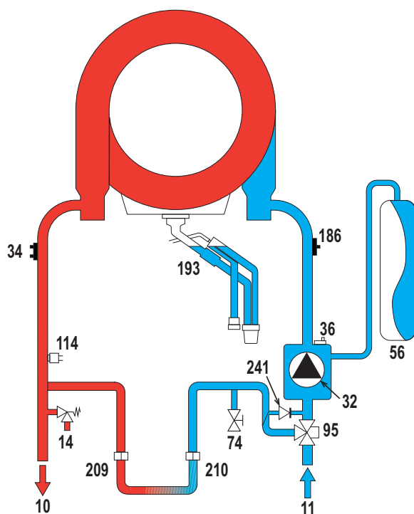
рис. 56- Гидравлический контур
