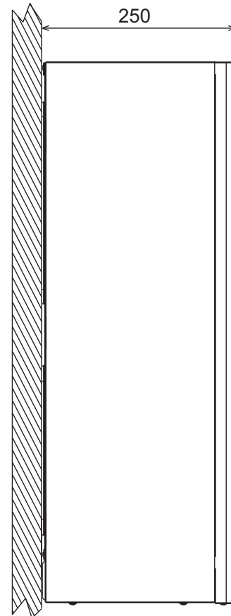
fig. 50 - Vista laterale
