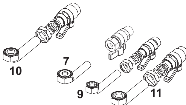
рис. 18- Гидравлический комплект
