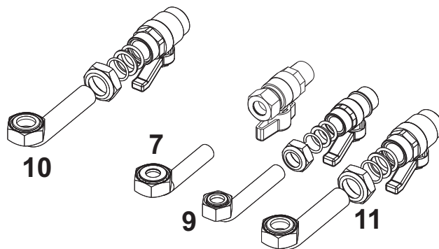
fig. 18 - Kit idraulico
