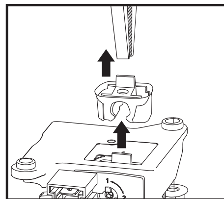
рис. 37- Замена газовой диафрагмы
