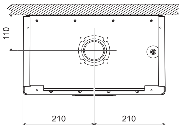
fig. 51 - Vista dall'alto
