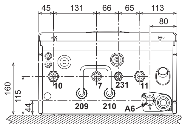
fig. 52 - Vista dal basso
