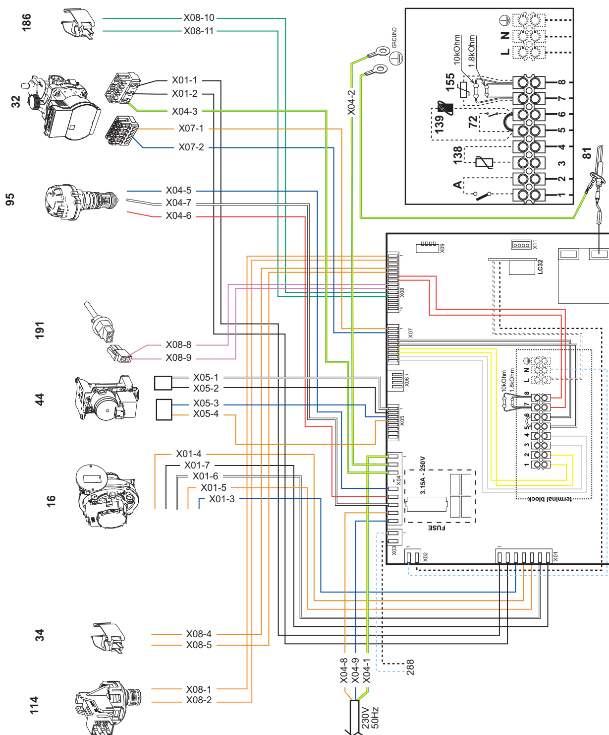
рис. 58- Электрическая схема
