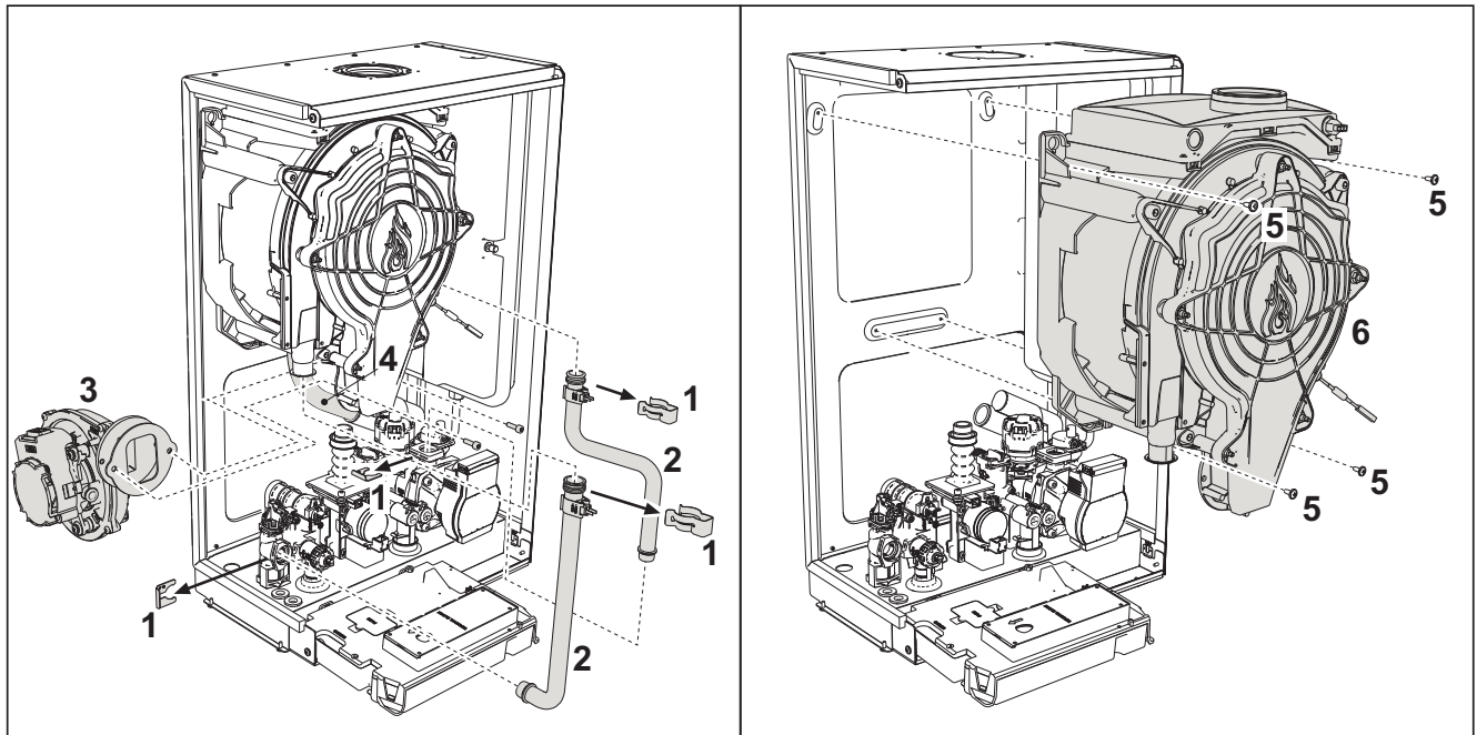
рис. 41- Основной теплообменник
