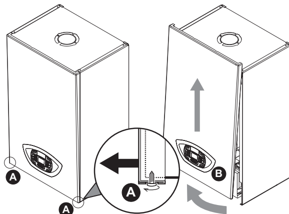
fig. 34 - Apertura pannello frontale
